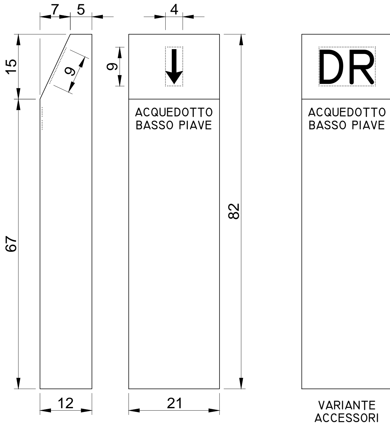
DETTAGLIO SCRITTE
